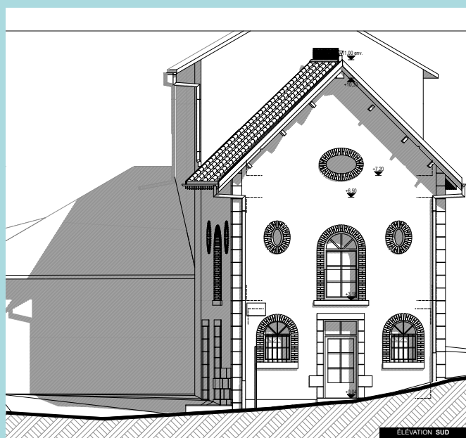
PLAN - Élévation SUD
