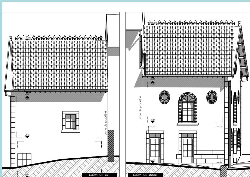
PLAN - Élévations EST - OUEST
